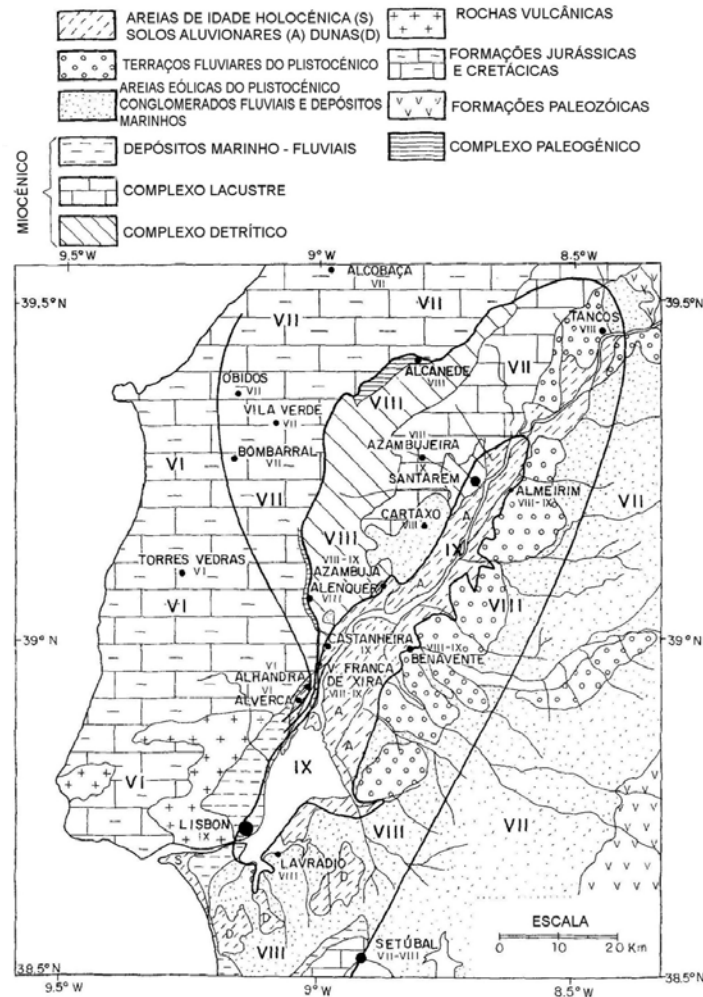
Figura 3 Mapa de isossistas do sismo de 1531, com informação geológica sobreposta
