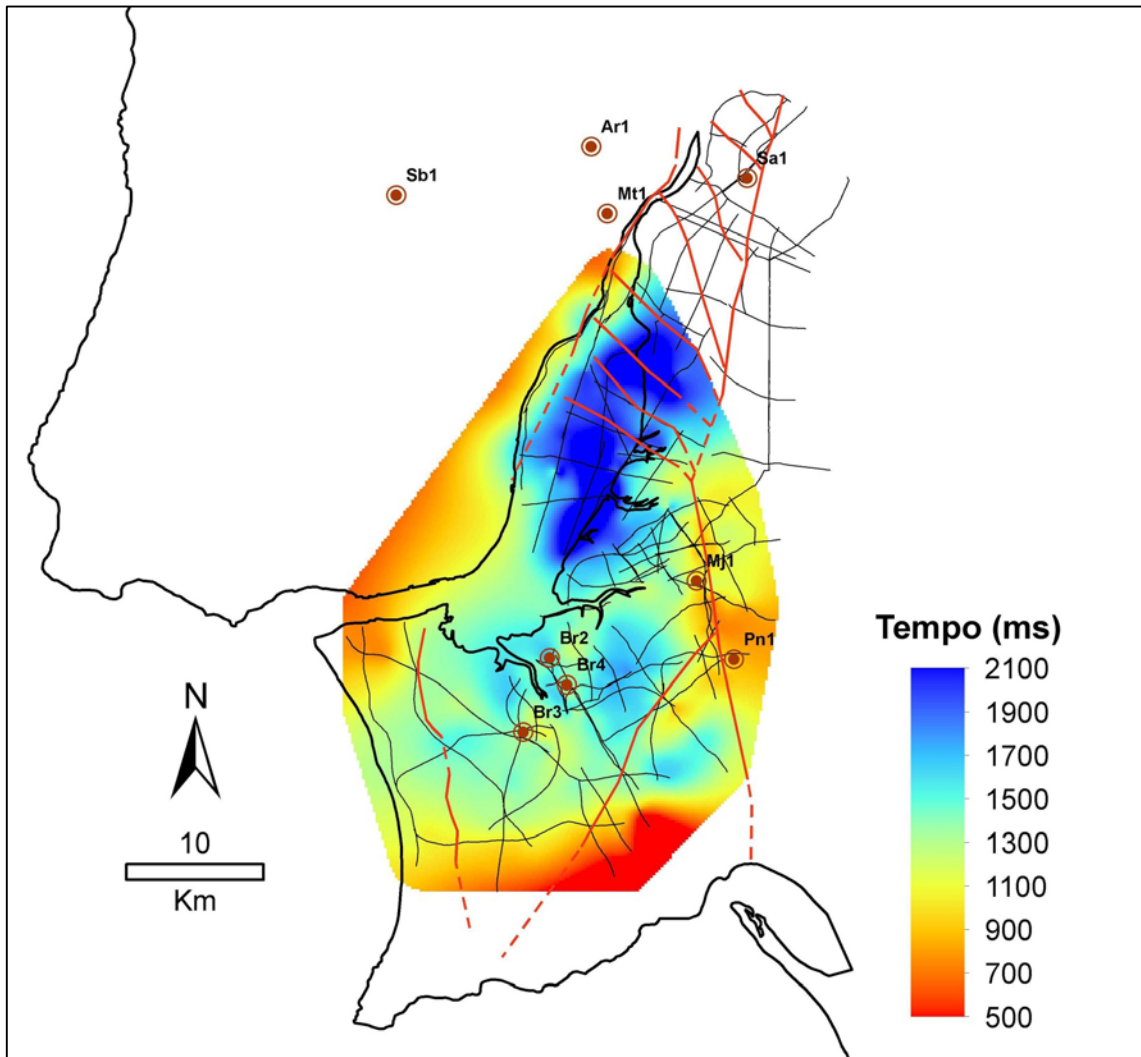
C. - Mapa do horizonte do topo aproximado da Formação de Montejuízo. As linhas a preto sobre a grelha indicam a localização dos perfis de sísmica de reflexão utilizados na interpolação. As linhas a vermelho indicam as falhas que afectam o horizonte. Os pontos a castanho indicam a localização dos furos profundos. Do lado direito da figura a escala de cores indica a variação da profundidade em tempo (ms) do horizonte.
