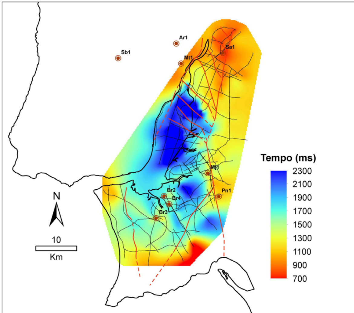
B. Mapa do horizonte do topo aproximado da Formação de Candeeiros-Brenha. As linhas a preto sobre a grelha indicam a localização dos perfis de sísmica de reflexão utilizados na interpolação. As linhas a vermelho indicam as falhas que afectam o horizonte. Os pontos a castanho indicam a localização dos furos profundos. Do lado direito da figura a escala de cores indica a variação da profundidade em tempo (ms) do horizonte.
