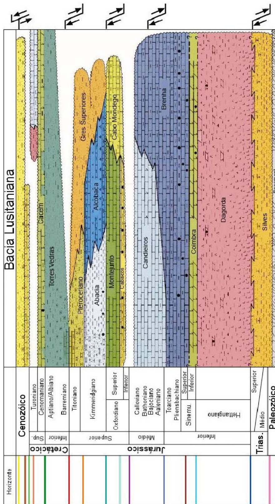
Figura 9 Unidades litoestratigráficas da Bacia Lusitaniana. À direita, estão marcadas (sob a forma de setas) as principais fases tectónicas, que condicionaram as seqüências (modificado de Rasmussen et al., 1998).
