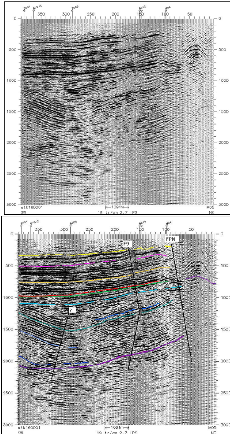
Figura 48 Imagem superior: Perfil M5, do lado direito (do shotpoint 1 a 100) é possível observar a deformação causada pela tectónica salina. Na imagem inferior é também possível observar o perfil interpretado com a marcação das falhas FPN e F9.
