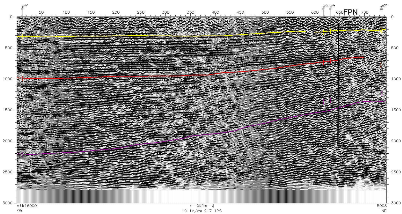
Figura 38 Evolução da deformação longo da FPN. Os perfis que atravessam a falha (a azul) são de Norte para Sul: B38NE, M03, Mo5, 221 e B008. Escala horizontal indicada nos perfis. No perfil B38NE observa-se a deformação extensa (shotpoint ~100 a300) assinalada com um rectângulo branco.
